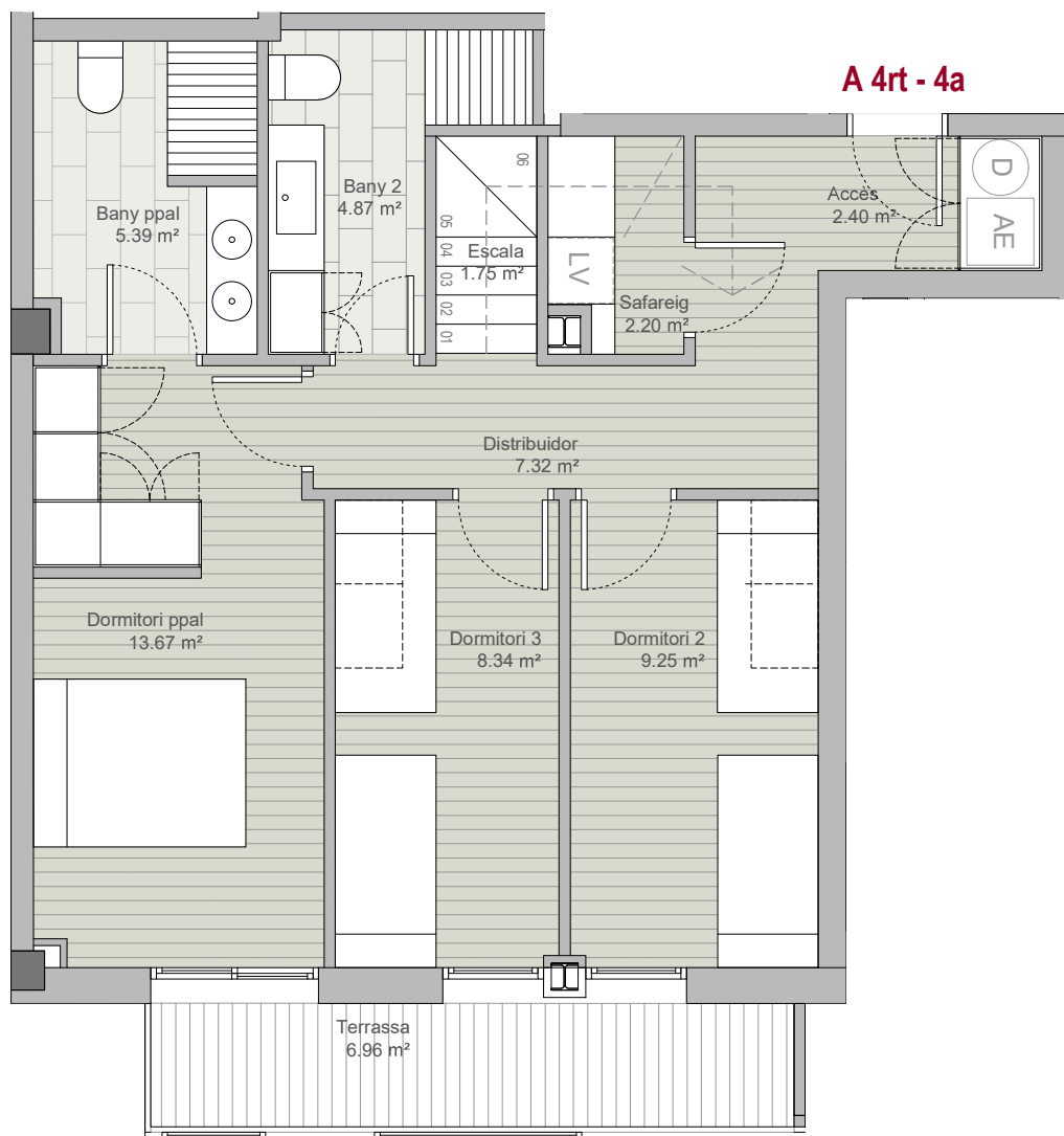
DÚPLEX ÀTIC - PLANTA INFERIOR
