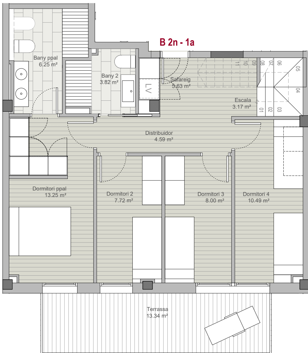
DÚPLEX ÀTIC - PLANTA INFERIOR
